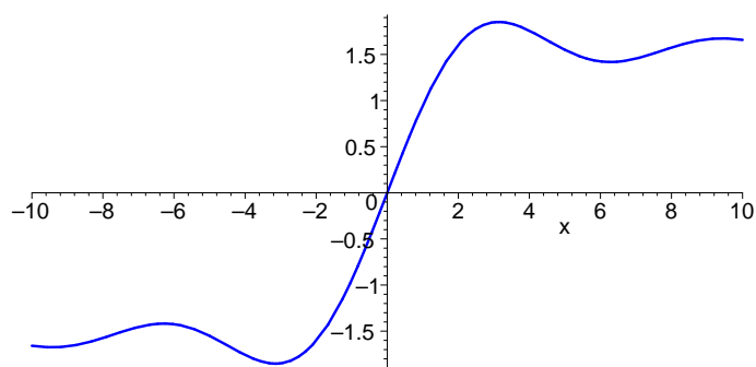
Der Integralsinus
