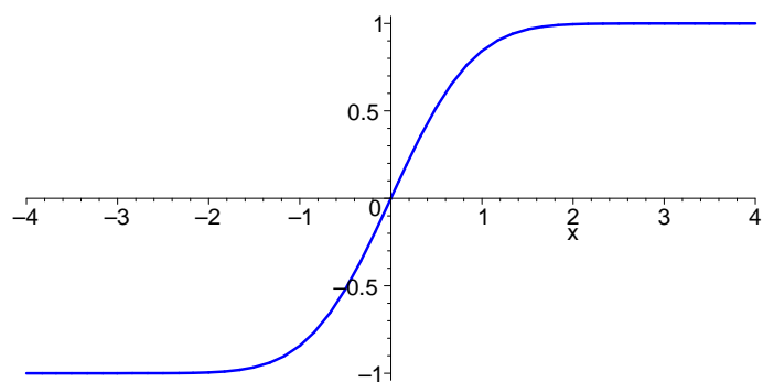
Die Fehlerfunktion
