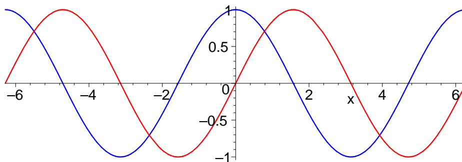
Sinus und Kosinus zwischen -2\pi und 2\pi
