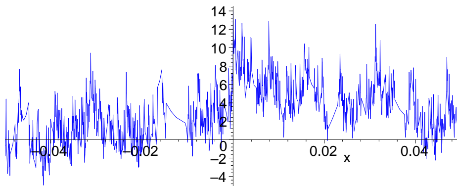
Vergrößerung um den Faktor zwanzig
