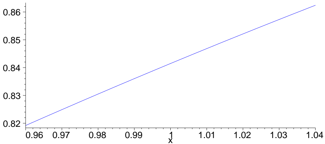
Nach noch einer Vergrößerung sieht die Funktion praktisch linear aus
