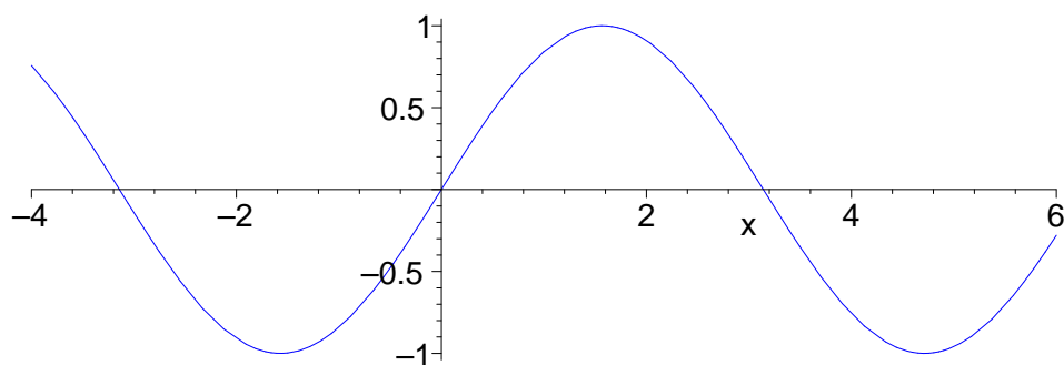
Graph der Funktion y = \sin x
