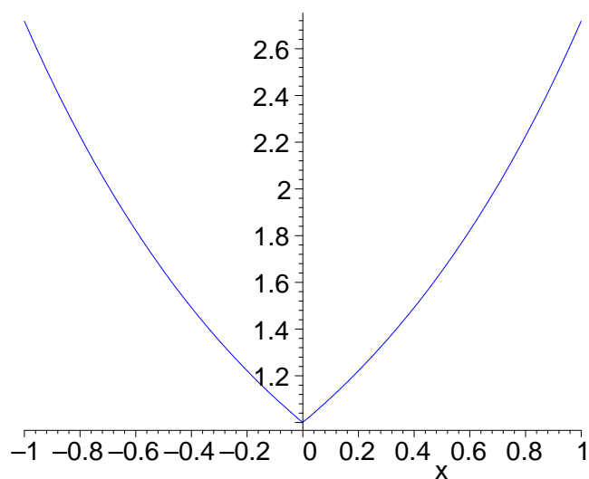
Graph der Funktion y = e^{|x|}
