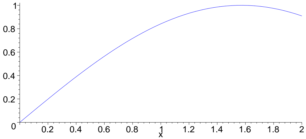
Vergrößerung um den Faktor fünf um (1, \sin(1))
