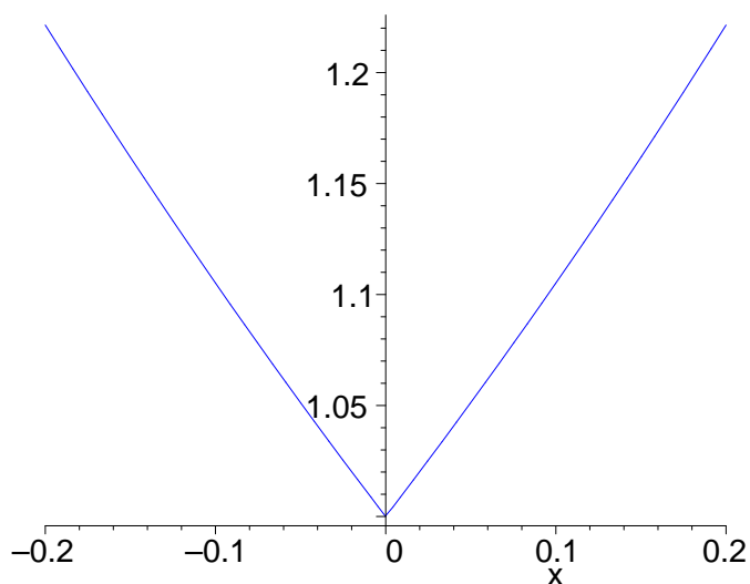
Vergrößerung um den Faktor fünf
