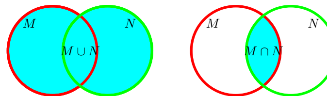
Die Vereinigung M \cup N
