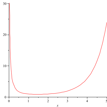
Die \Gamma -Funktion
