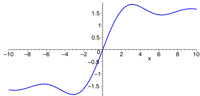
Der Integralsinus
