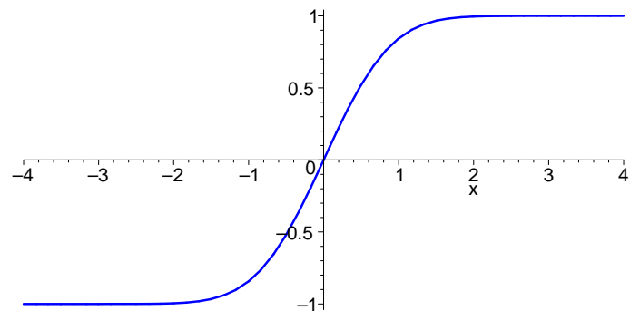
Die Fehlerfunktion
