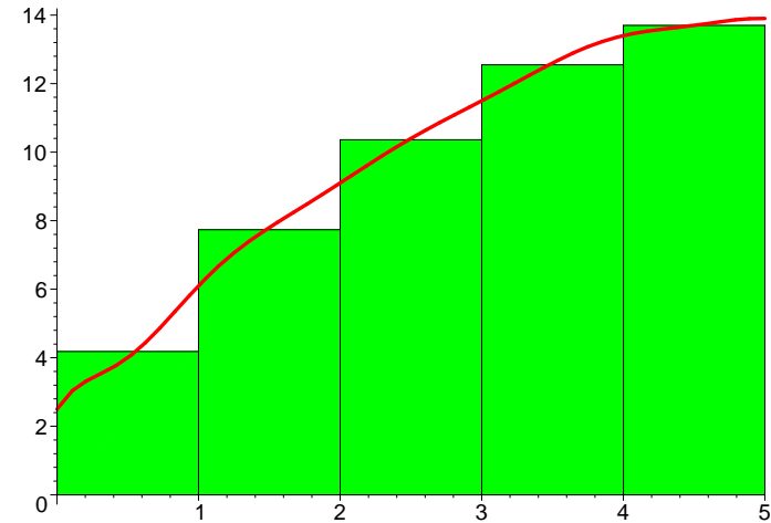
Die Fläche unter der Kurve ist gleich der Fläche der fünf Rechtecke
